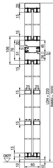
Navpični prerez
