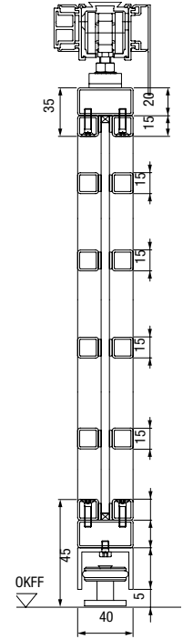
Navpični prerez
