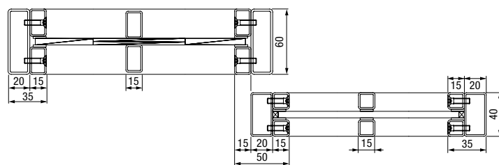
Vodoravni prerez 2-krilnih jeklenih podstrešnih vrat z obsvetlobo
