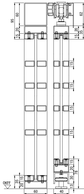
Navpični prerez 2-krilnih jeklenih podstrešnih vrat z obsvetlobo
