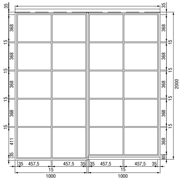
Navpični prerez 2-krilnih jeklenih podstrešnih vrat z obsvetlobo
