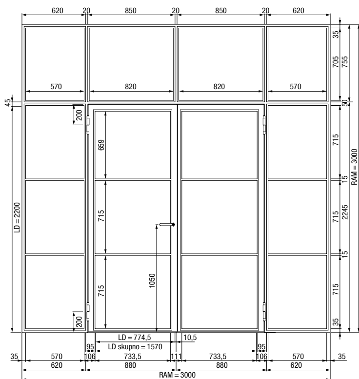
2-krilna jeklena podstrešna vrata z osvetlobami in nadsvetlobo
