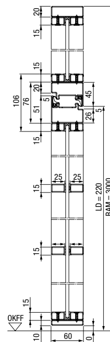
Navpični prerez 2-krilnih jeklenih podstrešnih vrat z nadsvetlobo
