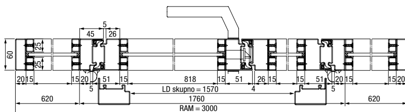
Vodoravni prerez 2-krilnih jeklenih podstrešnih vrat z osvetlobami
