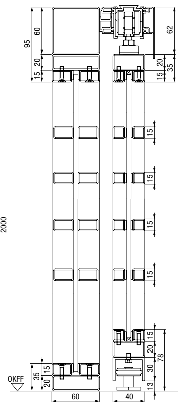
Navpični prerez 2-krilnih jeklenih podstrešnih vrat z osvetlobami
