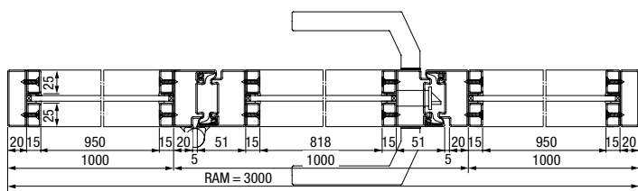
Vodoravni prerez 1-krilnih jeklenih podstrešnih vrat z obsvetlobami
