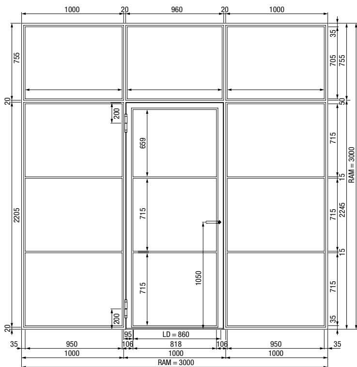
1-krilna jeklena podstrešna vrata z obsvetlobami in nadsvetlobo
