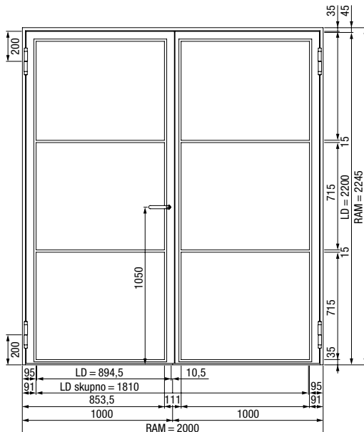
2-krilna jeklena podstrešna vrata
