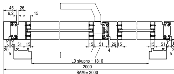
Vodoravni prerez 2-krilnih jeklenih podstrešnih vrat
