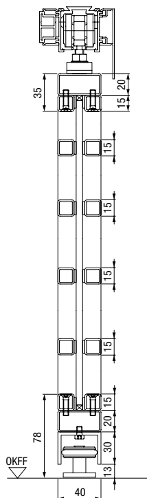
Navpični prerez 1-krilnih jeklenih podstrešnih vrat
