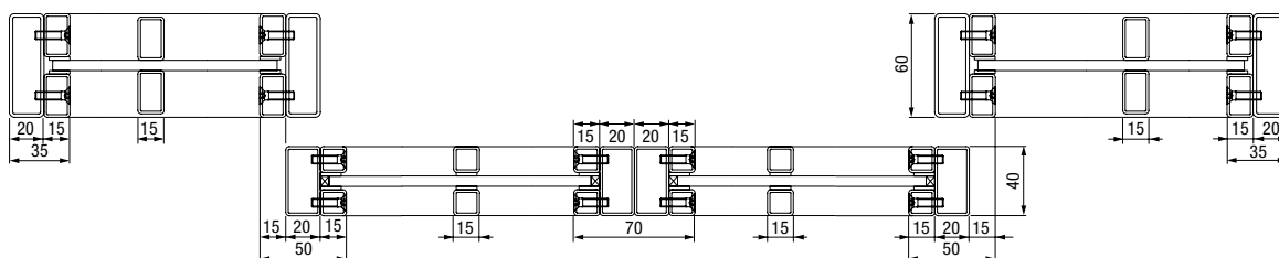
Vodoravni prerez 2-krilnih jeklenih podstrešnih vrat z osvetlobami
