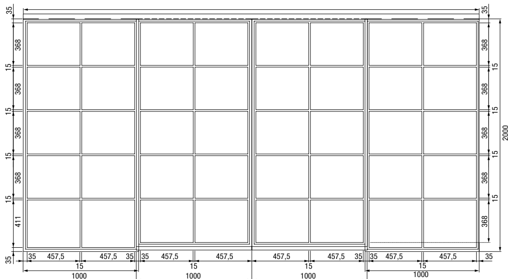
2-krilna jeklena podstrešna vrata z osvetlobami
