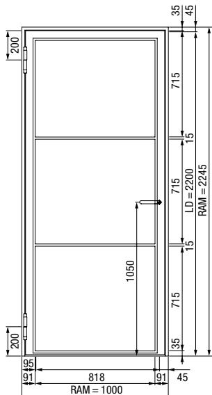
1-krilna jeklena podstrešna vrata
