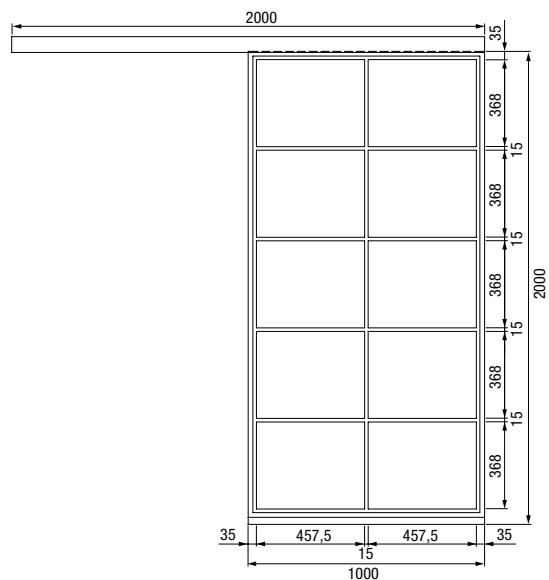
1-krilna jeklena podstrešna vrata
