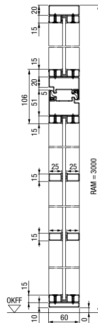
Navpični prerez 1-krilnih jeklenih podstrešnih vrat z nadsvetlobo
