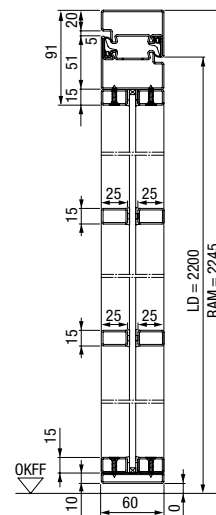
Navpični prerez 1-krilnih jeklenih podstrešnih vrat
