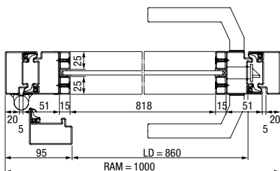
Vodoravni prerez 1-krilnih jeklenih podstrešnih vrat
