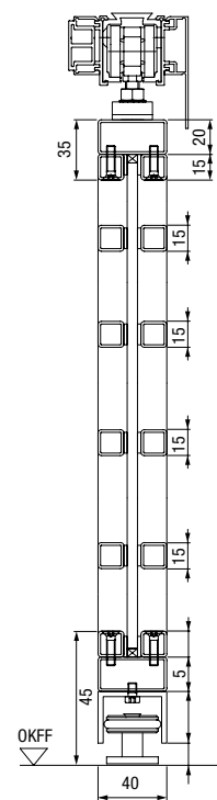
Navpični prerez
