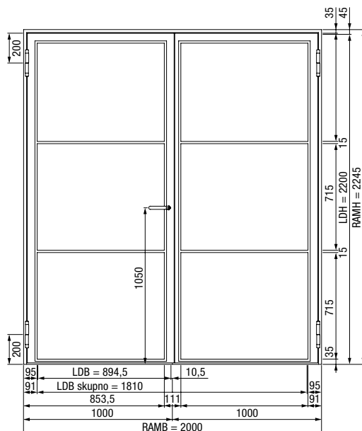
2-krilna vrata
