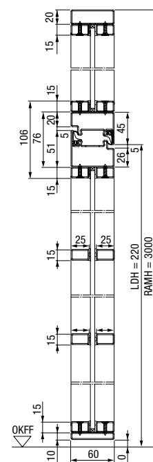
Navpični prerez
