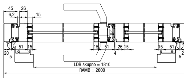
Vodoravni prerez 2-krilnih vrat
