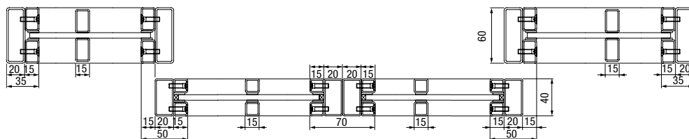
Vodoravni prerez
