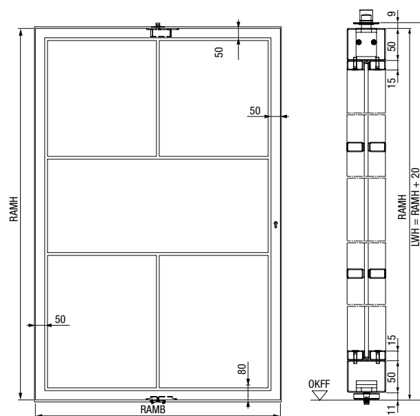
Vrtljiva vrata v standardni izvedbi s 50 mm širokim profilom okvirja in 50 mm visokim podnožjem, motiv 2
