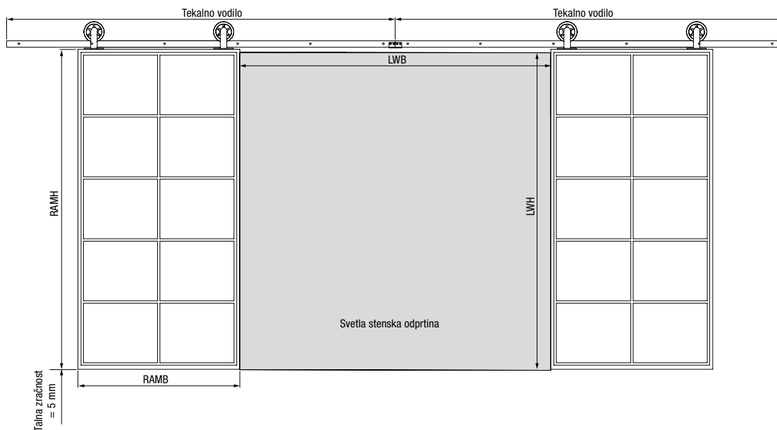
2-krilna retro podstrešna drsna vrata
