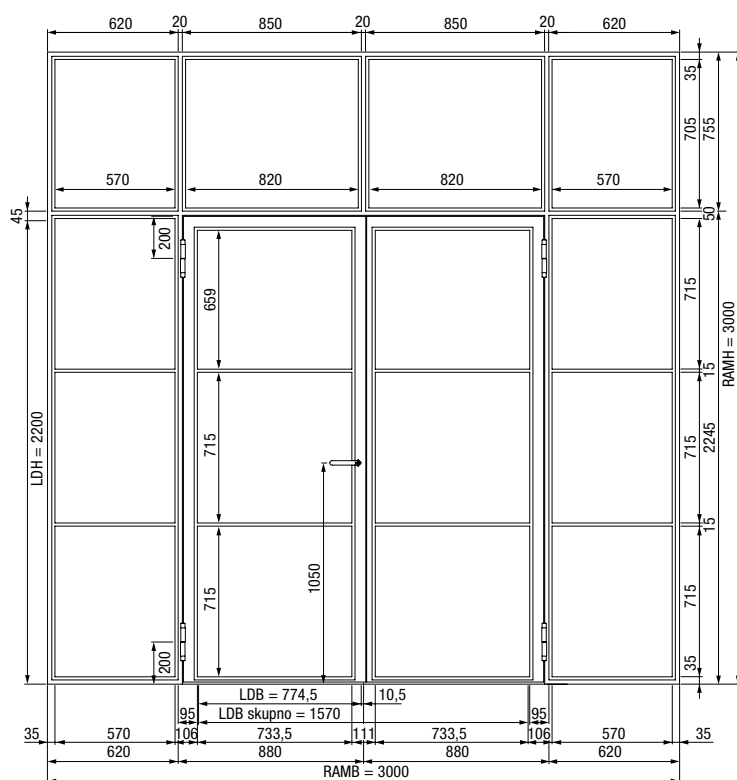
2-krilna vrata z osvetlobo in nadsvetlobo
