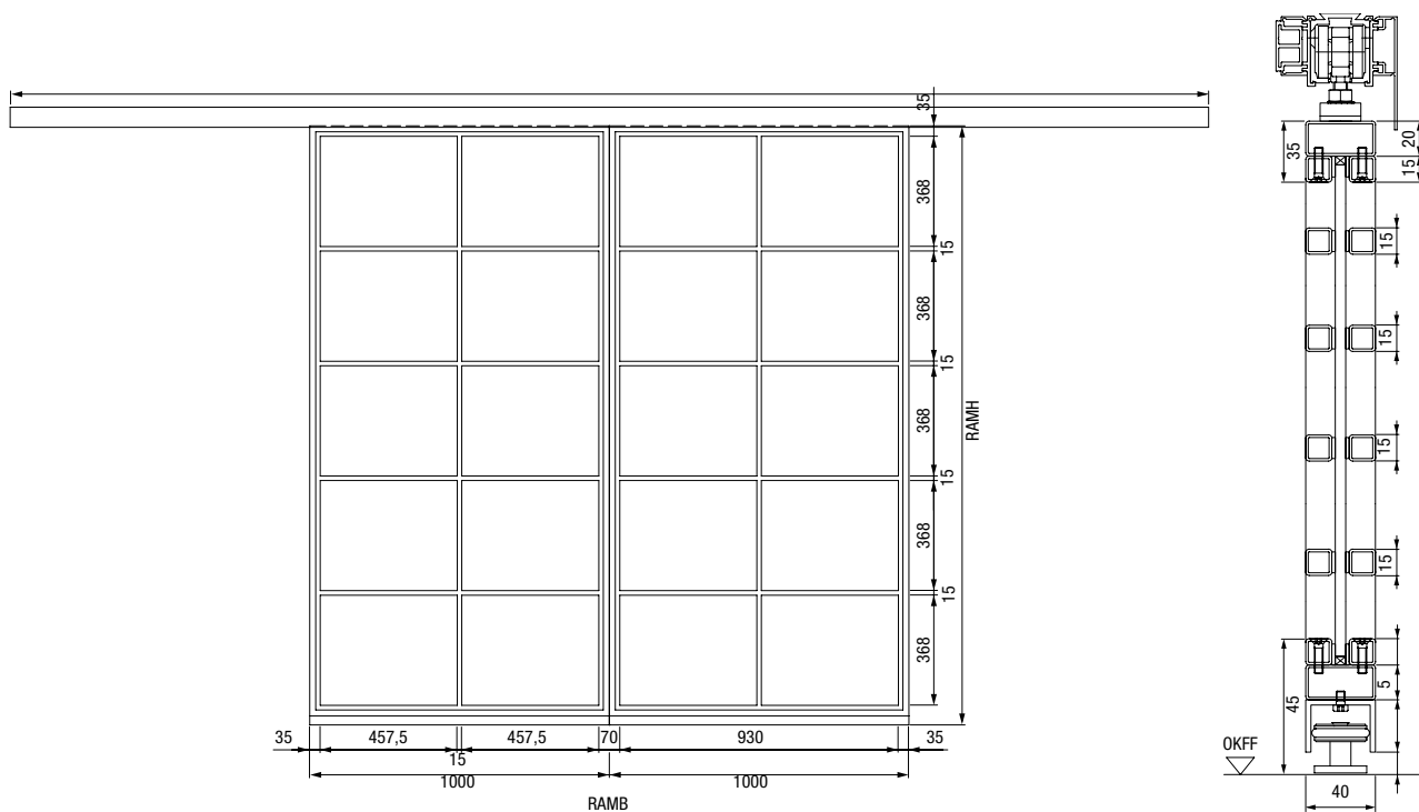
1-krilna drsna vrata
