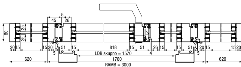
Vodoravni prerez
