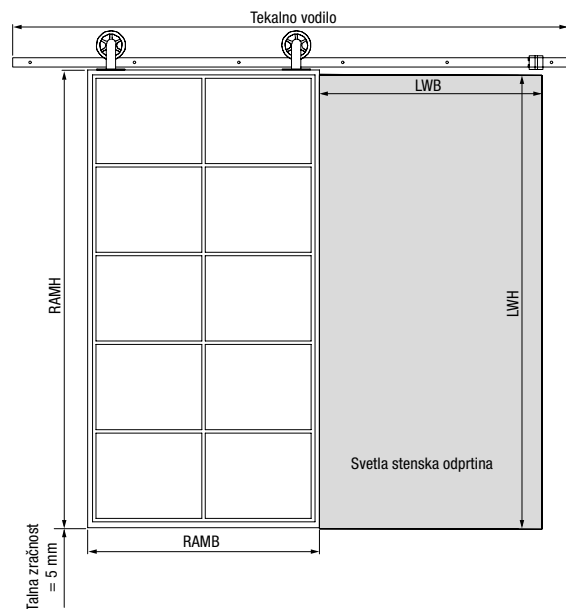
1-krilna retro podstrešna drsna vrata
