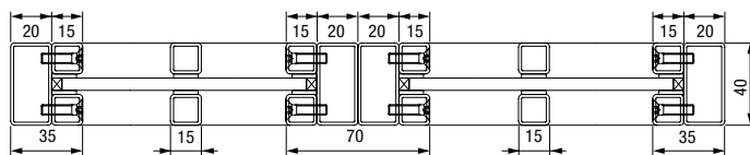
Vodoravni prerez
